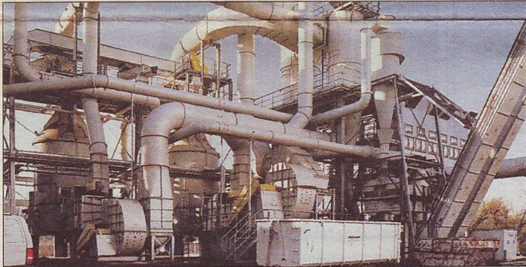
Viel Pneumatik im Umfeld der beiden Schwebesichter (links) und der Siebanlage (rechts) Fotos: H. Soiné und Dieffenbacher/Deinhard
